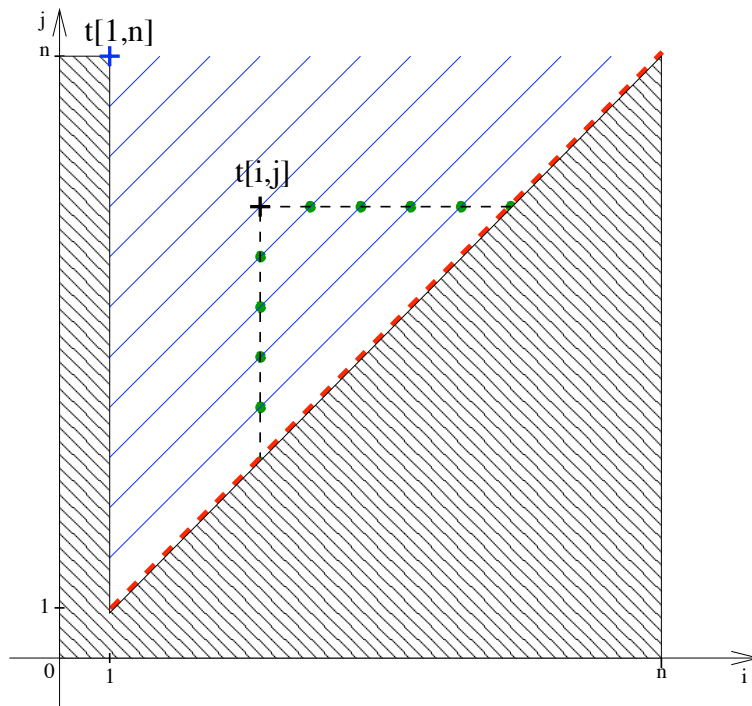
FIG. 2 – Diagramme (i, j) des valeurs à calculer par l'algorithme de résolution
