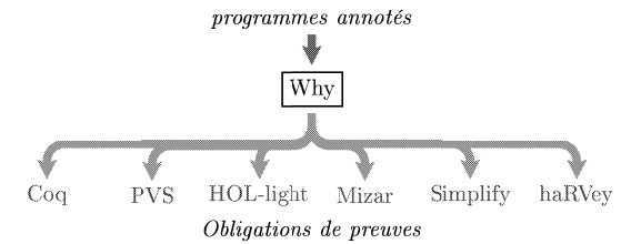
FIG. 8.2 – Approche multi-prouveur de Why
